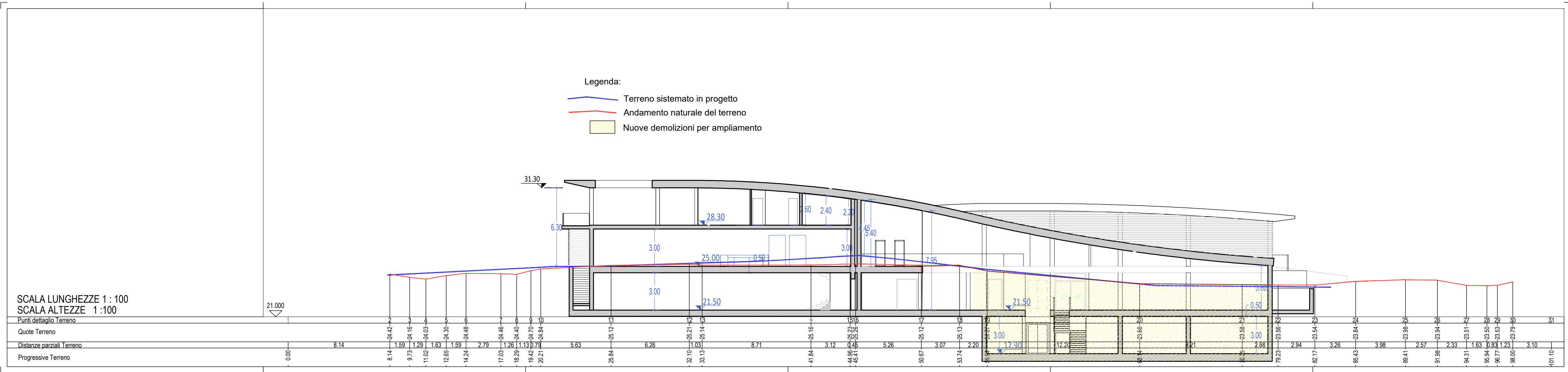
PROFILO LONGITUDINALE DEL TERRENO
